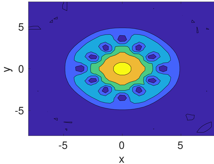
GPEvortex2D #2 , t = 15.000
